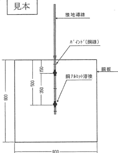
テルミット2点接続
