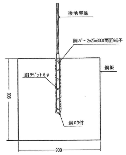
銅帯リベット止め後ロー付
